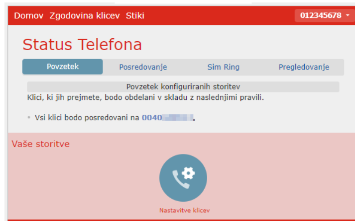
Slika 5: Nastavitve klicev
