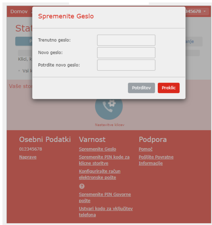
Slika 3: Sprememba gesla
