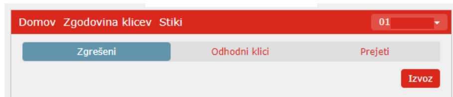
Slika 11: Zgodovina klicev
